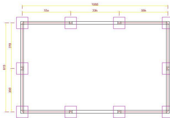
FONDATION
