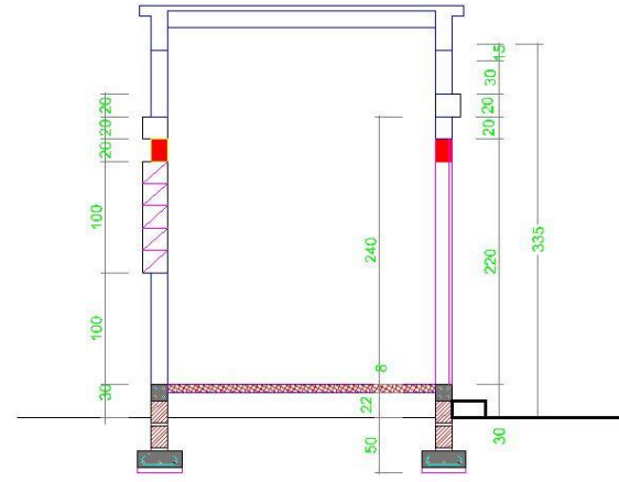
COUPE AA
