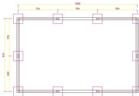
FONDATION
