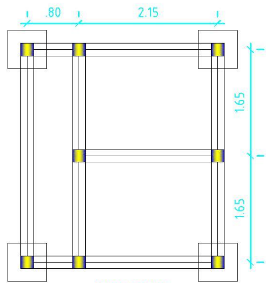
FONDATION
