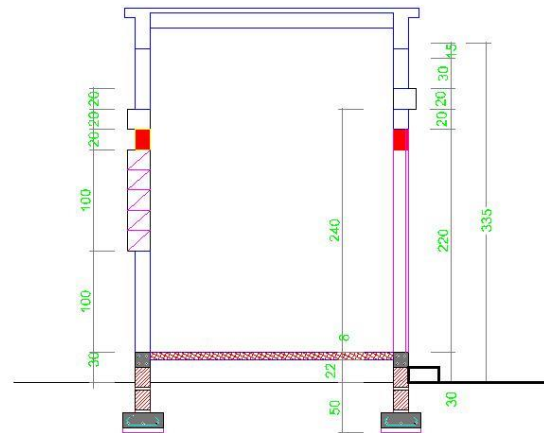
COUPE AA
