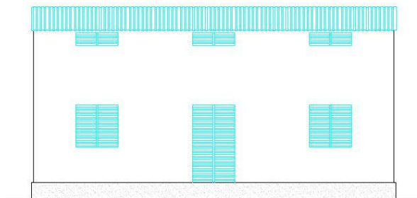
FACADE PRINCIPALE
