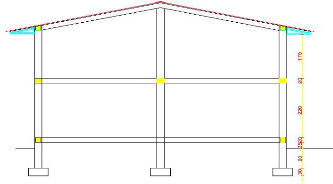
COUPE MAGASIN
