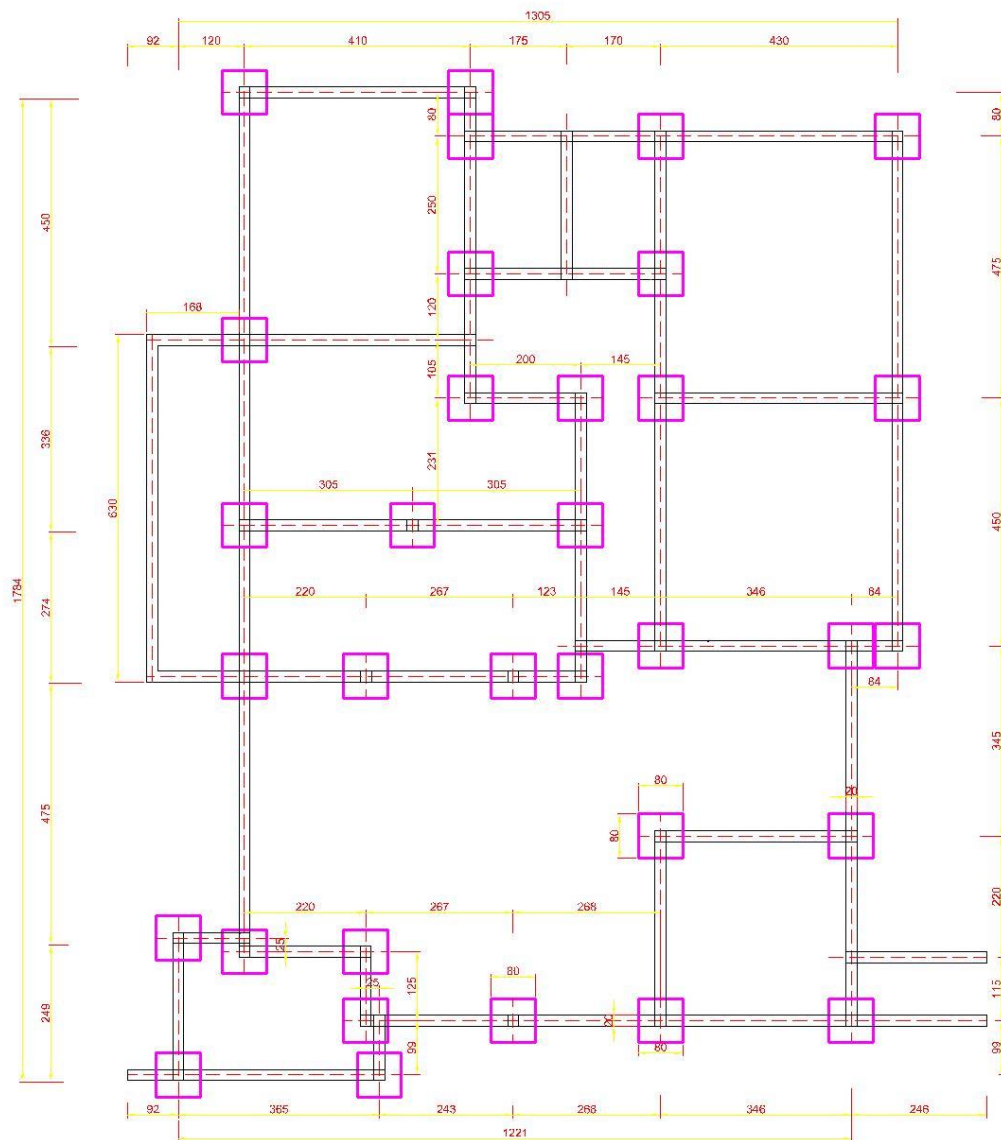
FONDATION
