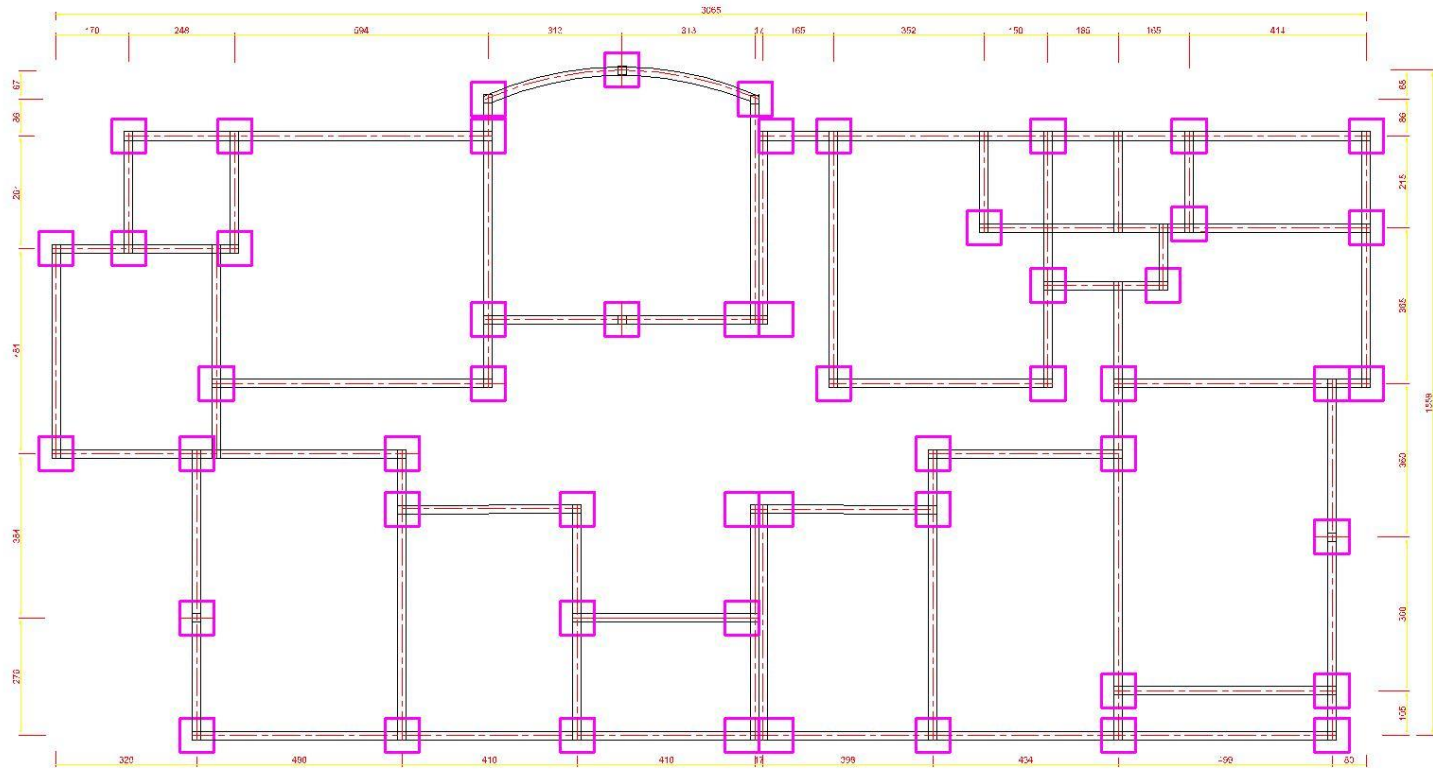
FONDATION
