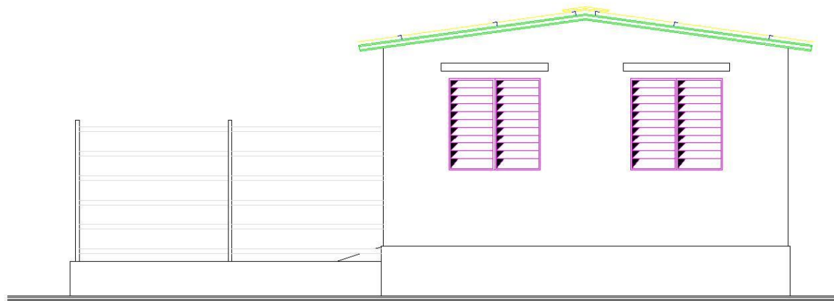
FAÇADE.LAT.DROITE
