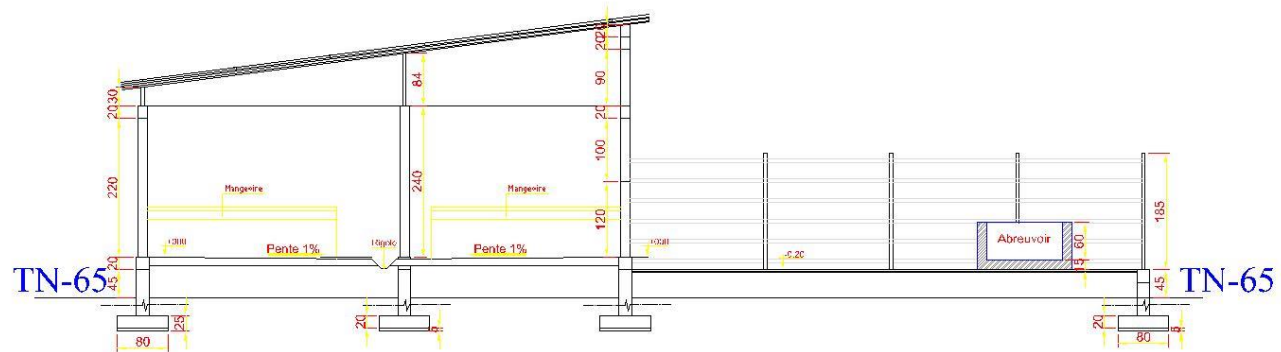
COUPE A-A
