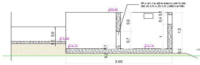
Coupe B-B
