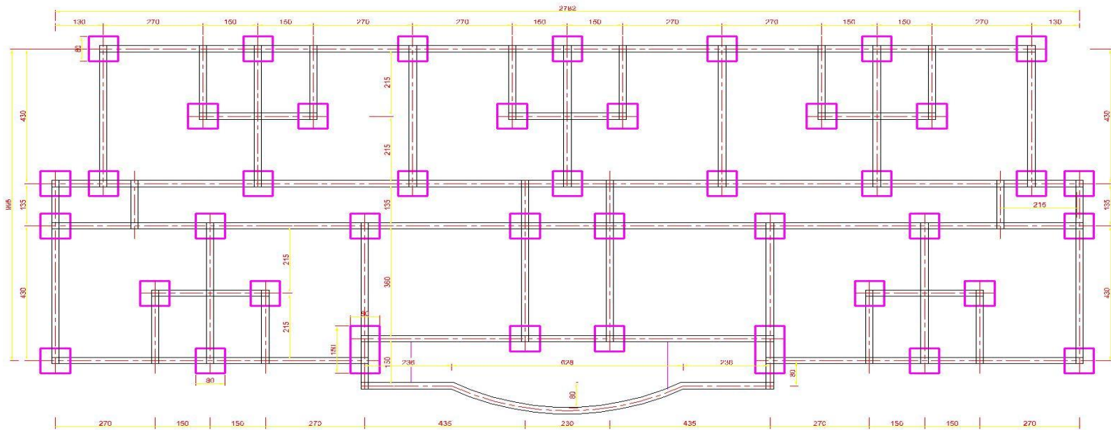
FONDATION
