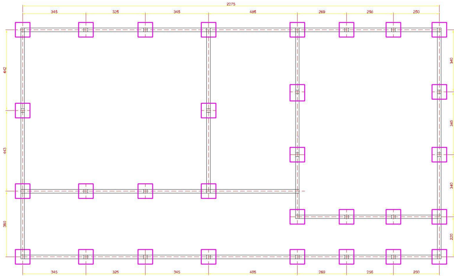
FONDATION
