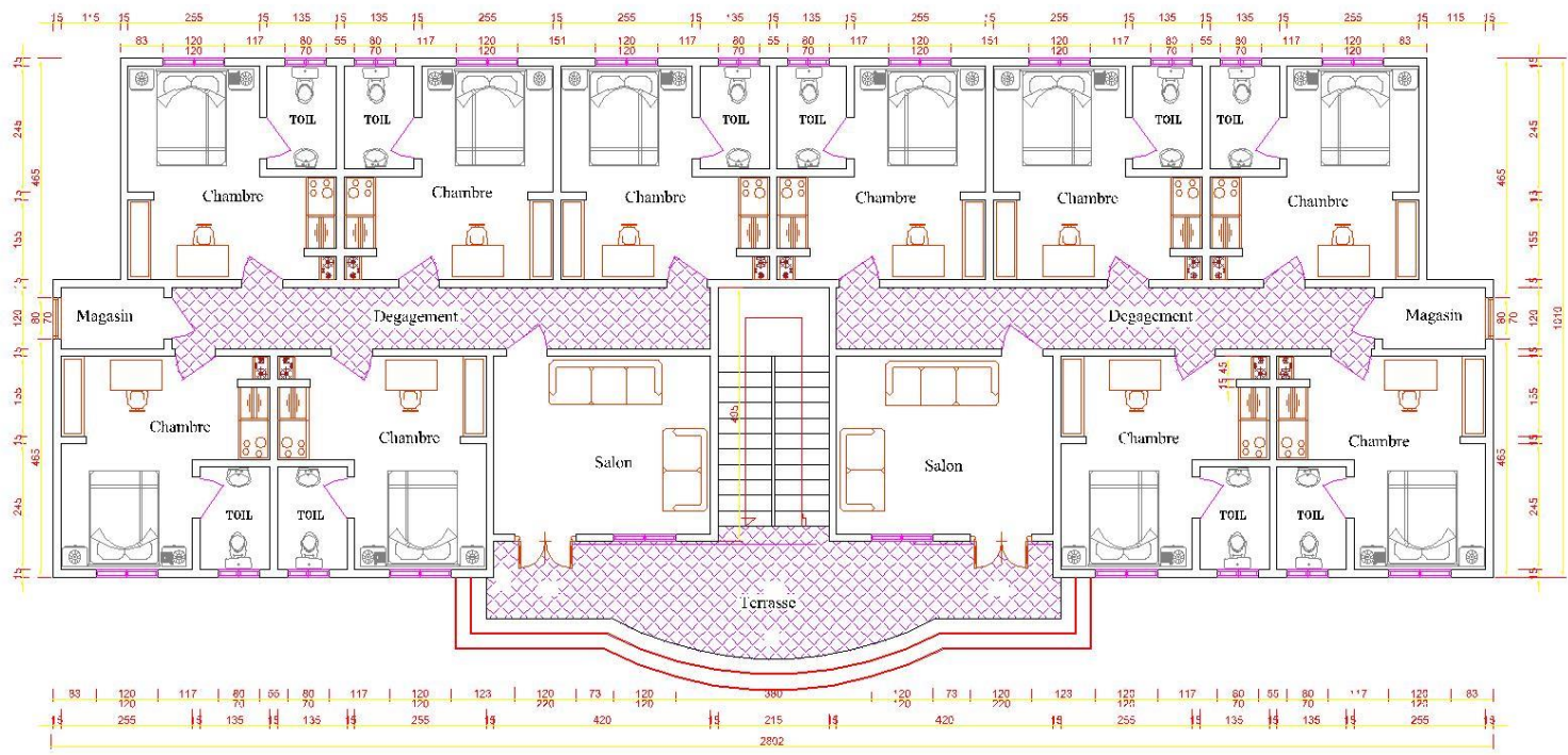
PLAN RDC
