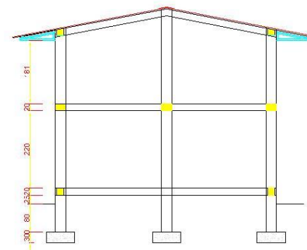
COUPE
