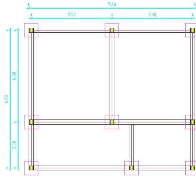
FONDATION
