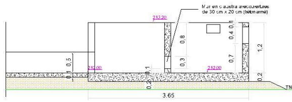
Coupe A-A
