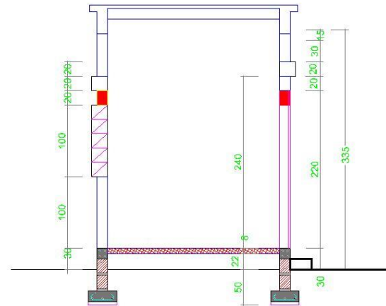
COUPE AA
