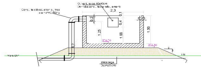
COUPE B-B
