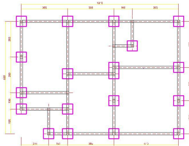
FONDATION
