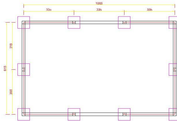
FONDATION
