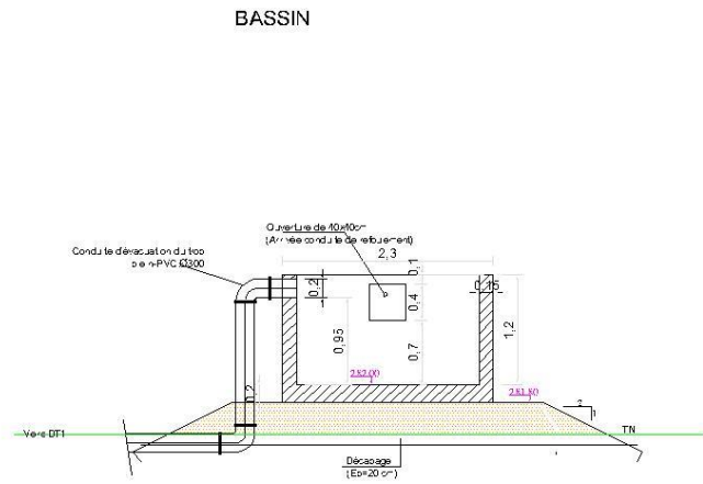
COUPE B-B
