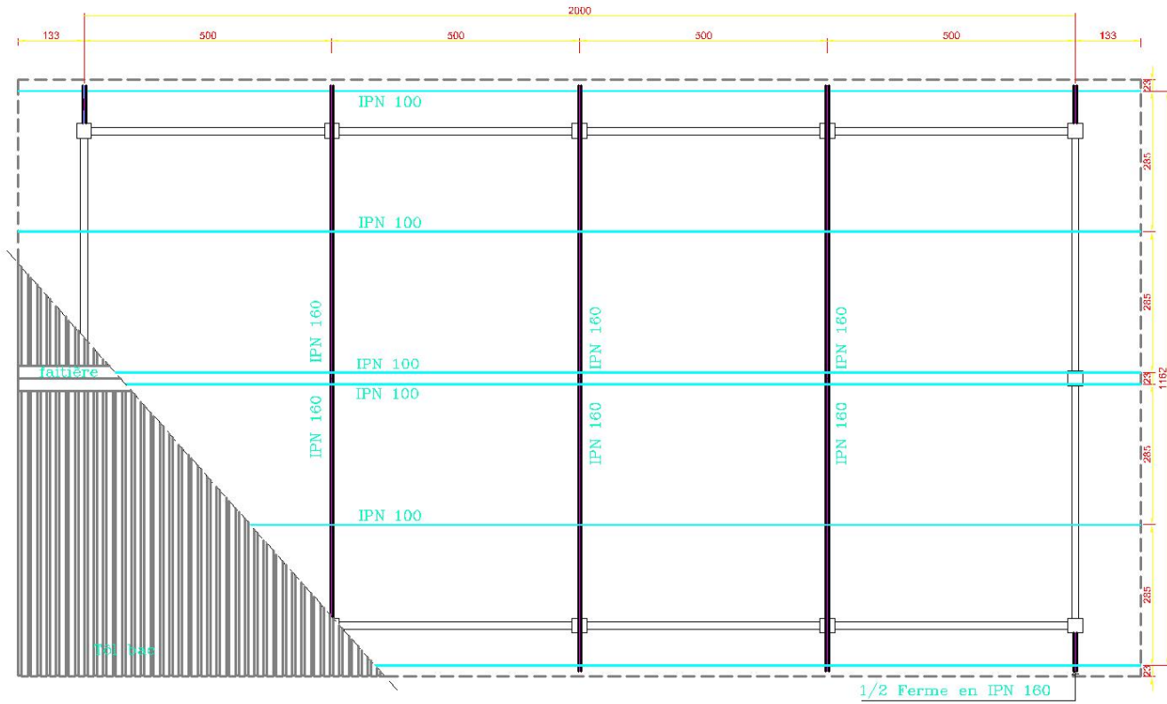
VUE EN PLAN DE LA TOITURE
