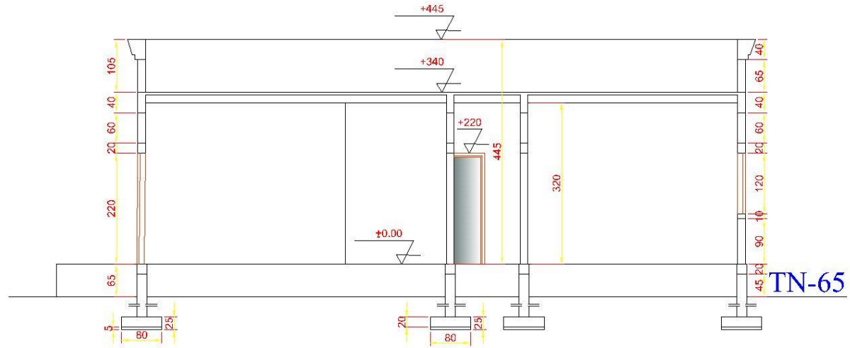
COUPE
