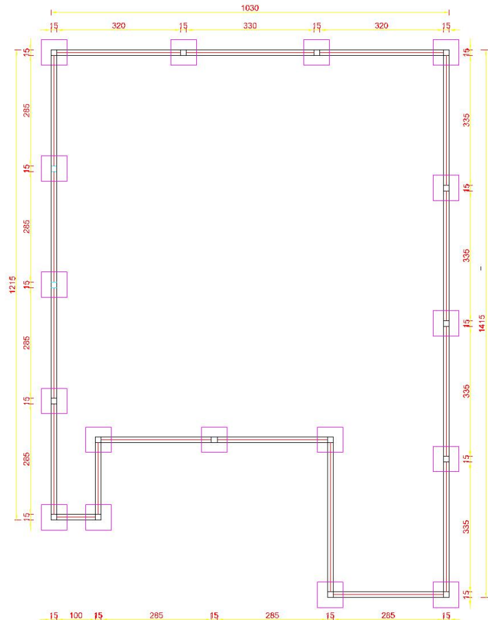
FONDATION
