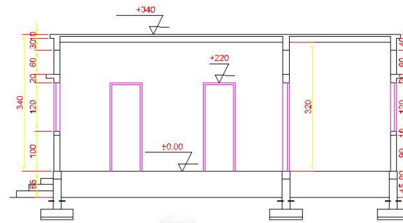
COUPE
