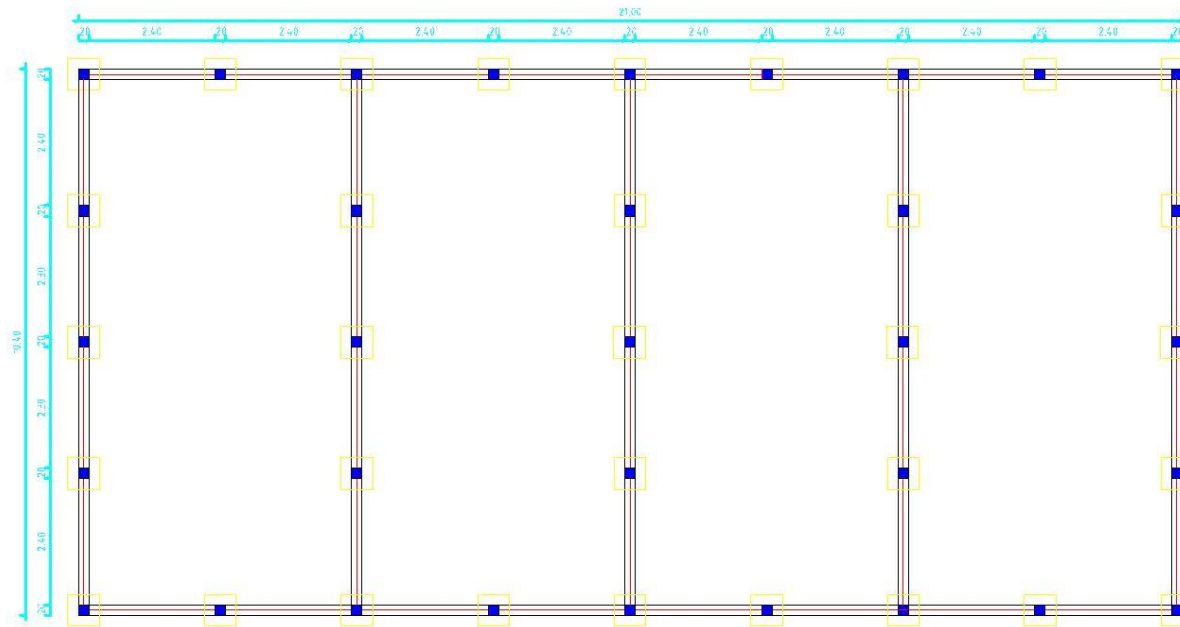
FONDATION
